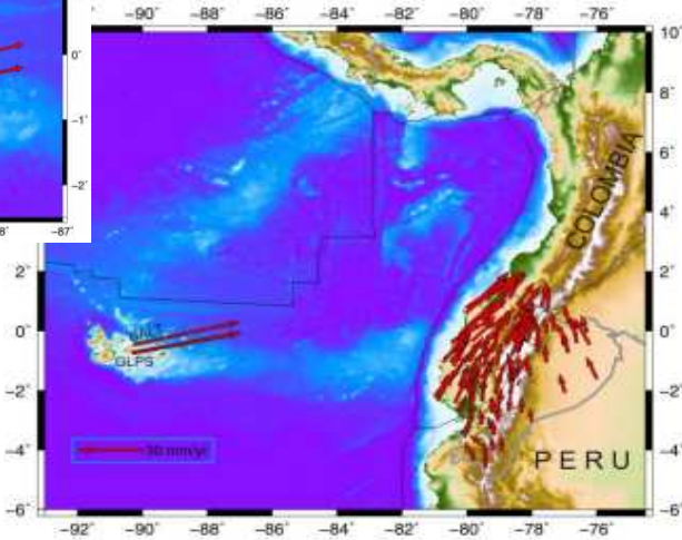
Figura No. 6: Campo de Velocidades del Ecuador. Fuente: Cisneros, D. and Nocquet, JM. (2011). CAMPO DE VELOCIDADES DEL ECUADOR, obtenido a través de Mediciones de Campañas GPS de los últimos 15 años y medidas de una Red GPS Permanente, IGM – IGEPN – GEOAZUR - IRD. Nice – France , 2011.
