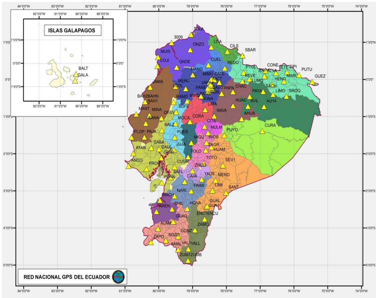
Figura No. 3: Red Nacional GPS del Ecuador - RENAGE
