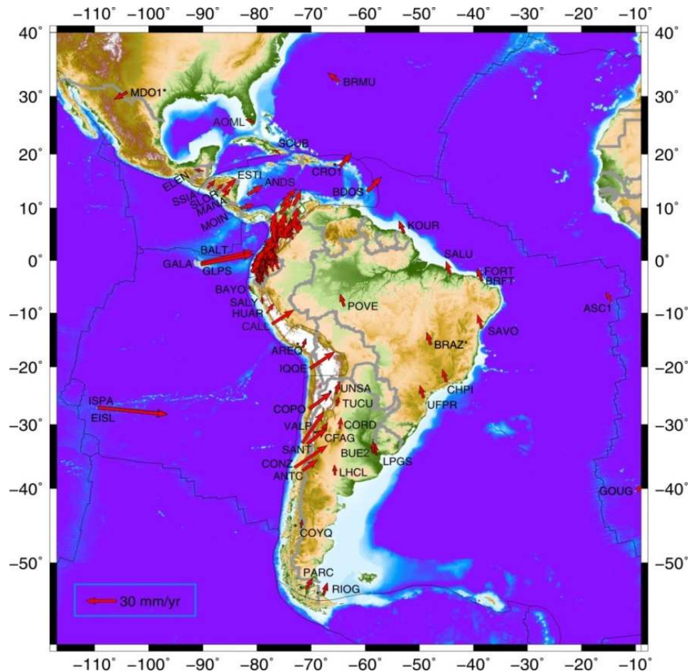
Figura No. 19: Campo de velocidad, estaciones permanentes SIRGAS_CON e IGS. Fuente: Cisneros, D. and Nocquet, JM. (2011). CAMPO DE VELOCIDADES DEL ECUADOR, obtenido a través de Mediciones de Campañas GPS de los últimos 15 años y medidas de una Red GPS Permanente, IGM – IGEPN – GEOAZUR - IRD. Nice – France , 2011.
